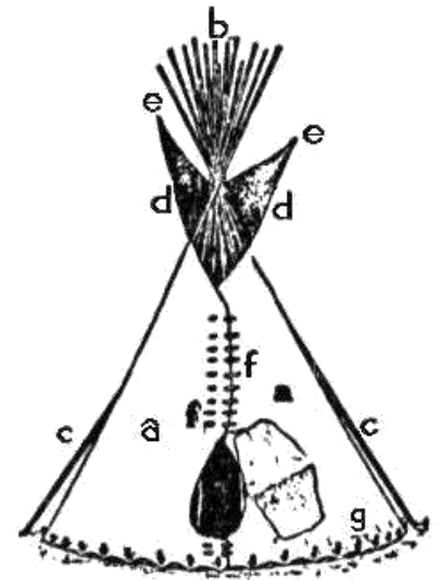
a huiden b palen c palen voor rookflappen d rookflappen e 'oren' f houten pinnen om de dekhuiden vast te zetten g houten haringen
